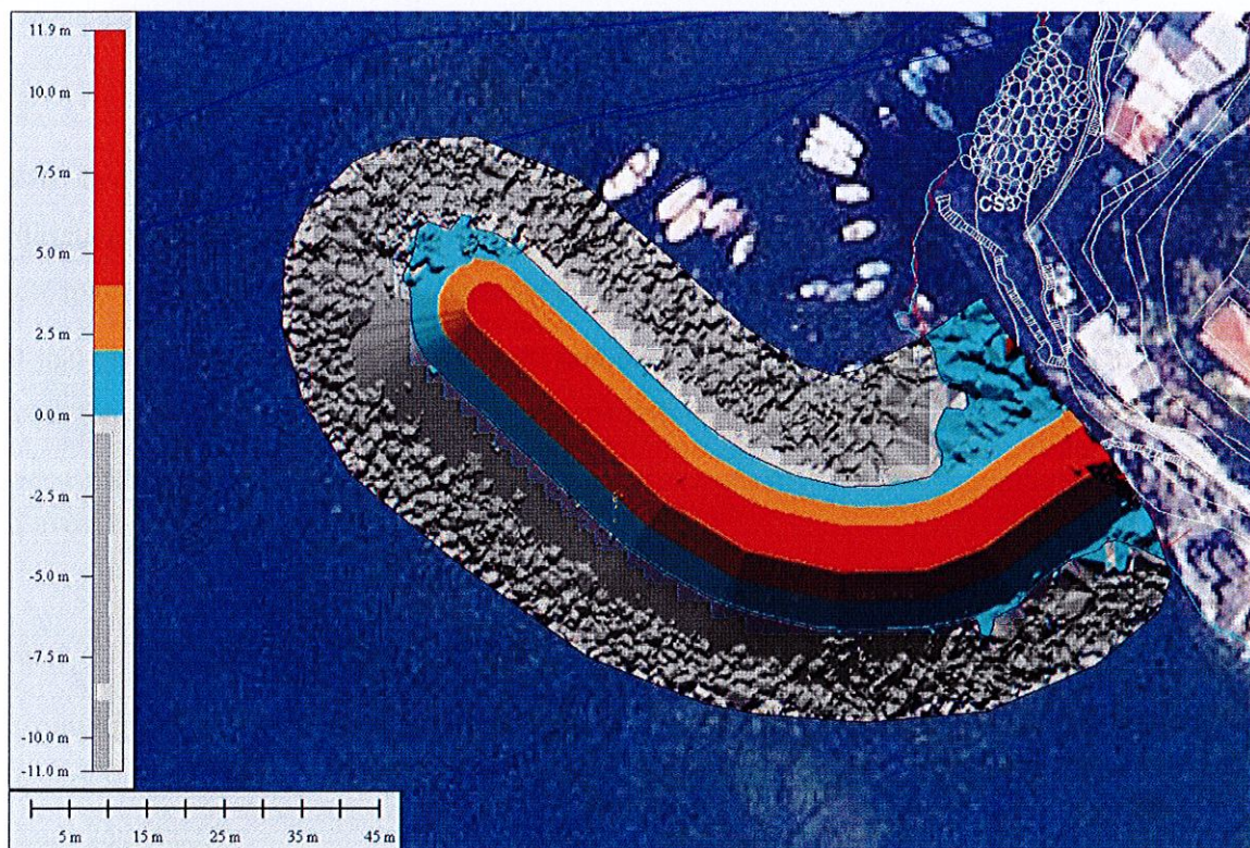
Figura 8 -rilievo Riomaggiore: rappresentazione grafica dello stato di progetto con colorazione per fasce di altezza
