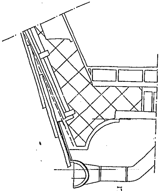
GRONDE E PLUVIALI IN RAME
