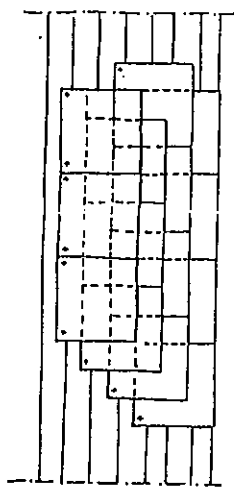
MANTO DI COPERTURA IN ARDESIA (59 x 59 x 0.51) cm SOVRAPPPOSTI DI 1/3, COLMI IN LATERIZIO
